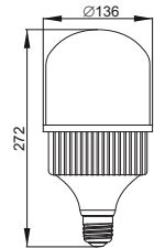
Рисунок 35 – Лампа LED-HP, 80 Вт, 100 Вт, цоколь E40
