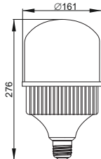
Рисунок 34 – Лампа LED-HP, 65 Вт, цоколь E40
