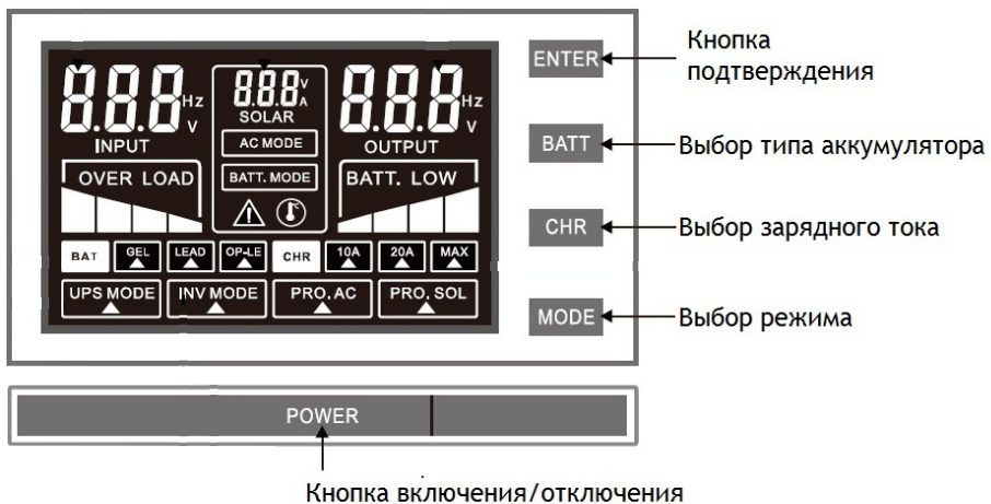
Рис.3 Панель управления
