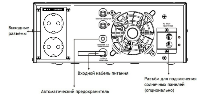
Рис.1 Задняя панель
